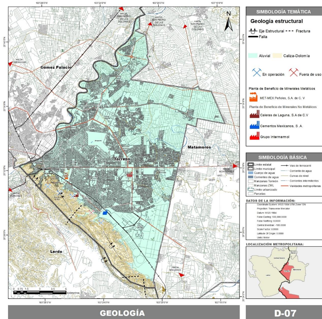
Mapa 7. Geología
