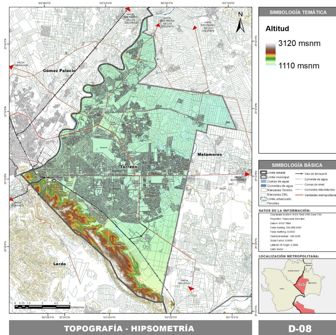
Mapa 8. Hipsometría
